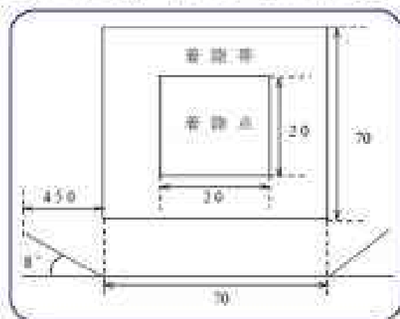
(d-2) 大型機 (UH-47 及び V-107) の場合《応急》
