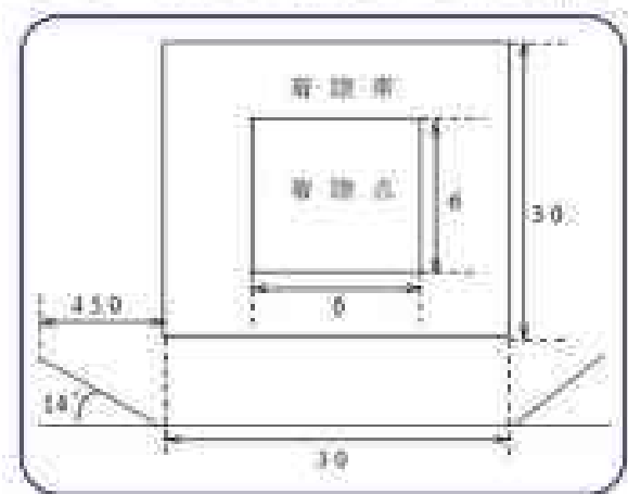
(b-2) 中小型機 (OH-1) の場合《応急》
