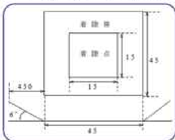
(a-1) 大型機（LH-60）の場合（標準）
