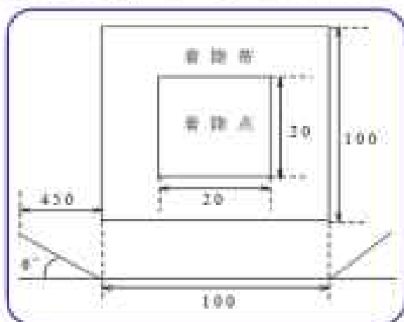
(a-1) 大型機（H-47 及び H-107）の場合（標準）
