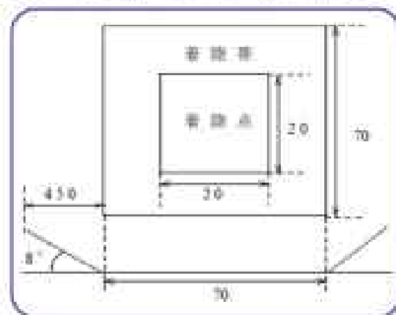
(a-2) 大型機（H-47 及び H-107）の場合（応急）
