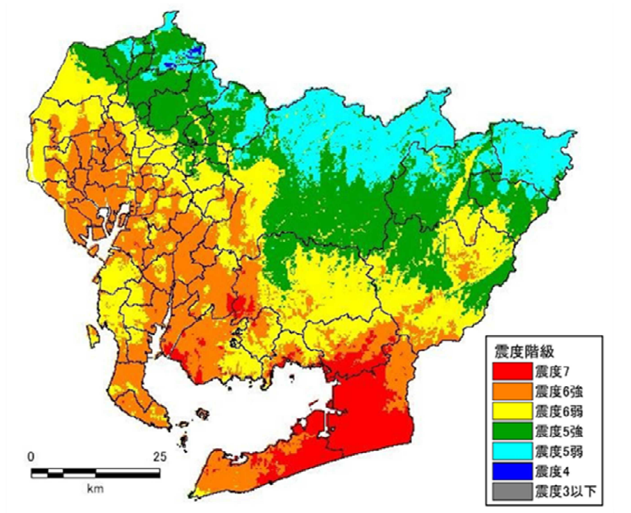
○ 理論上最大モデル 東側ケース 震度分布図
