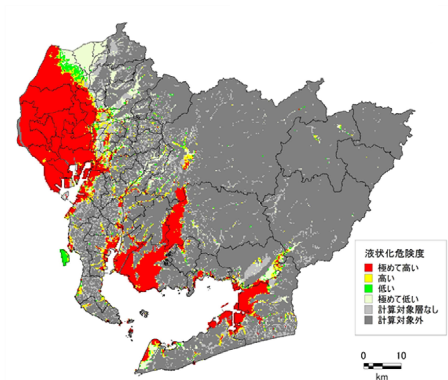
○ 理論上最大モデル 東側ケース 液状化危険分布図
