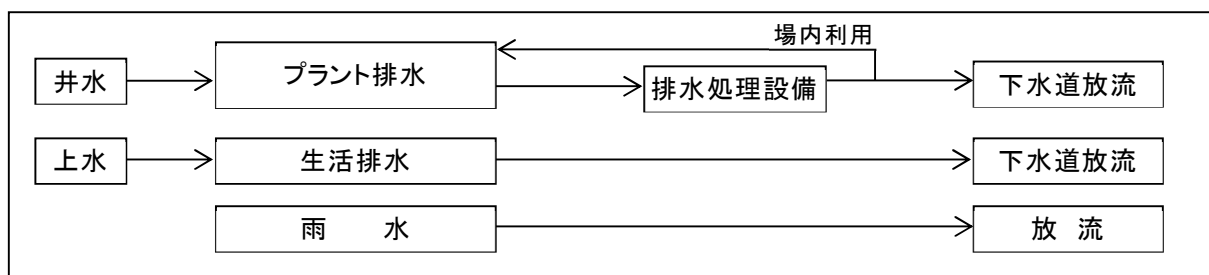
図2.2.3 給排水フロー図
