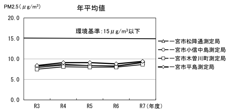
図 3.1.11 微小粒子状物質（年平均値）の経年変化
