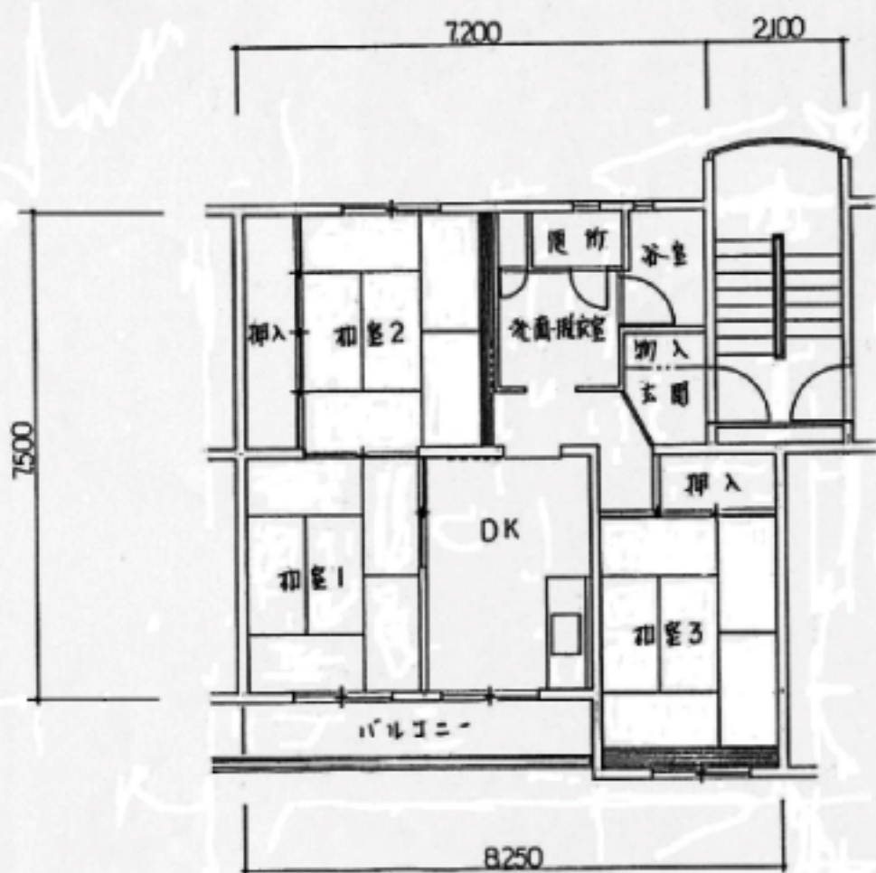
矢合用地 3~5 棟平面図 SC=1/100
