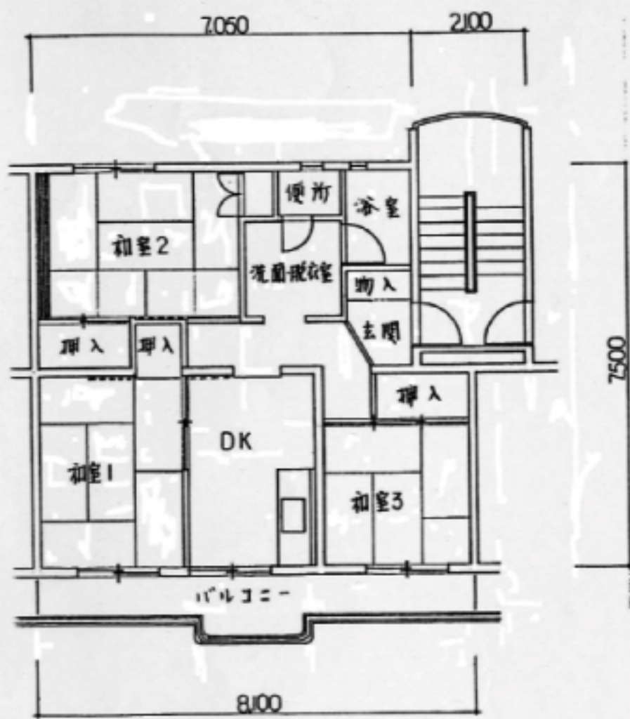
矢合用地 1.2 棟平面図 SC=1/100
