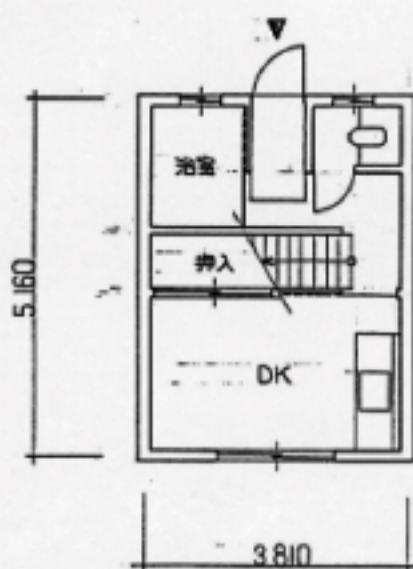
西島団地16棟平面図
