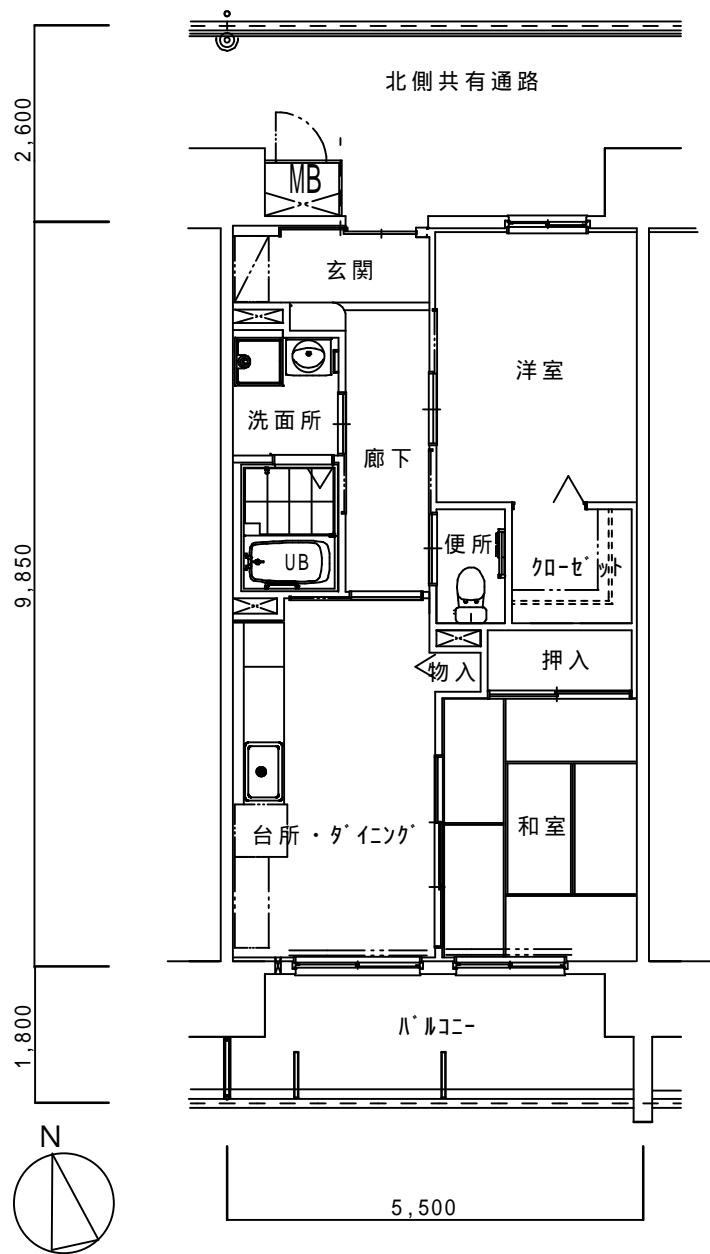
A - 1タイプ 高齢者住宅 2DK (54.17m 2 )
