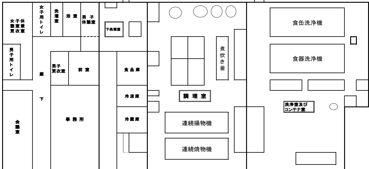
旧平和町学校給食センター調理場内配置図
